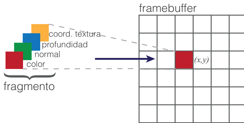
Figura 4: Representación de un fragmento.
