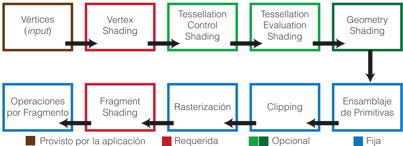
Figura 2: Una representación simplificada del pipeline gráfico de OpenGL mostrando cada una de sus etapas.
