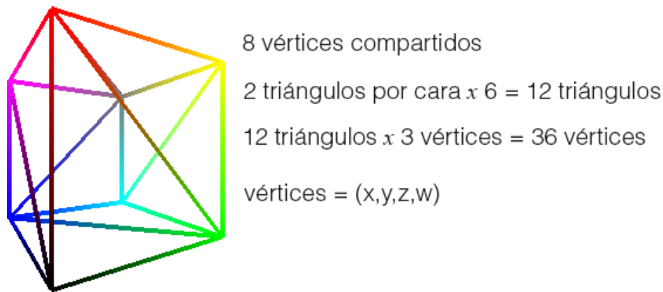
Figura 5: Cubo de ejemplo con su especificación geométrica.
