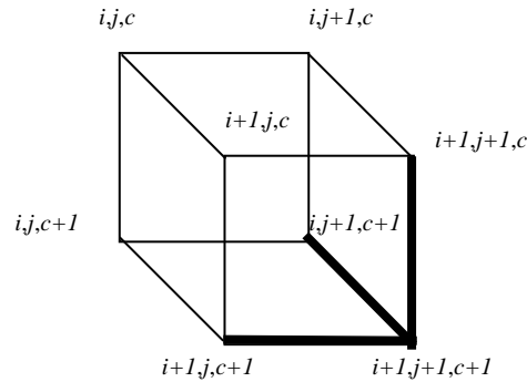
Figura 4.1: Aristas asociadas a IV[c,i,j]
