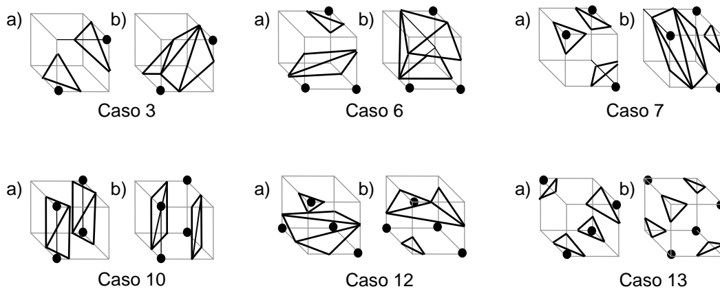
Figura 3.5: Los seis patrones ambiguos
