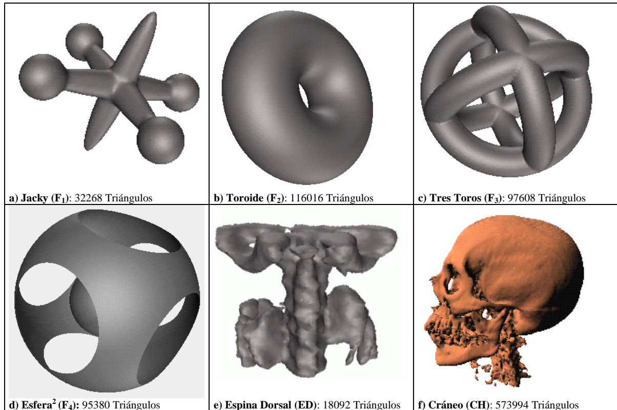
Figura 5.1: Imágenes resultantes de la triangulación
