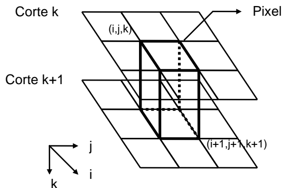
Figura 3.1: Voxel
