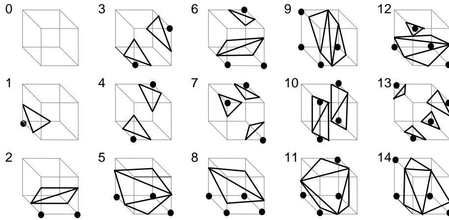
Figura 3.4: Los 15 patrones y su triangulación
